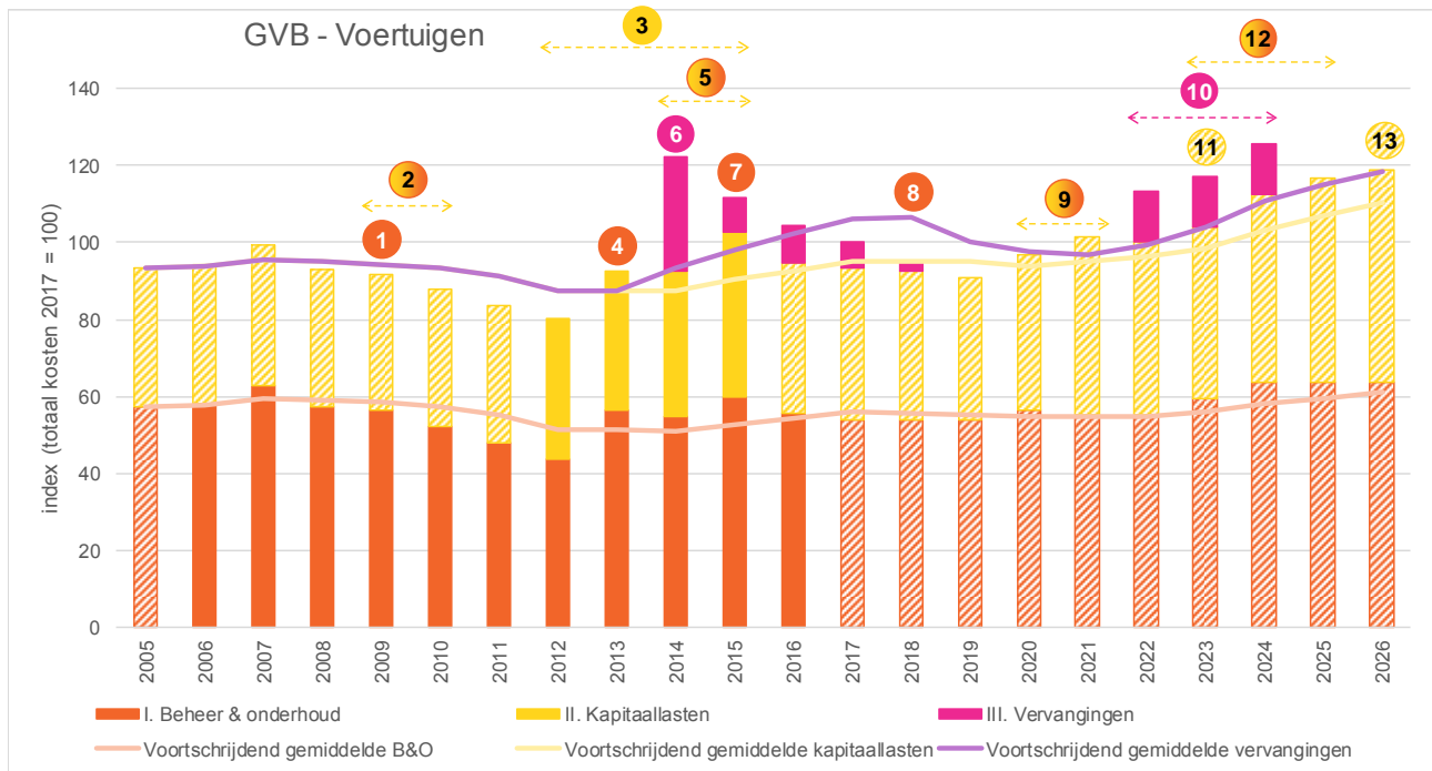
Figuur 15: BOV-kosten GVB voertuigen (2005-2026) 9
